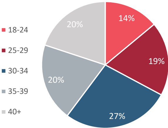
Nhóm tuổi
